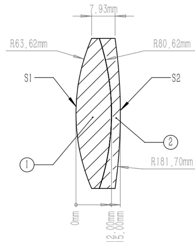
剖面 A-A
