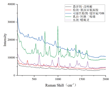
不同剂型农药的拉曼光谱
