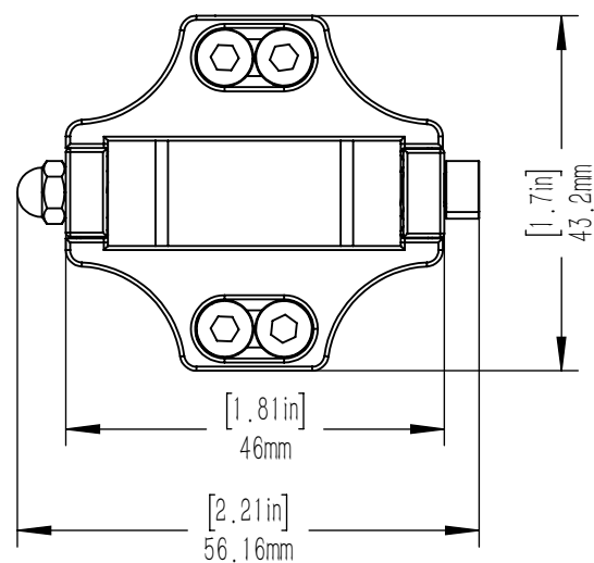
视图 A
